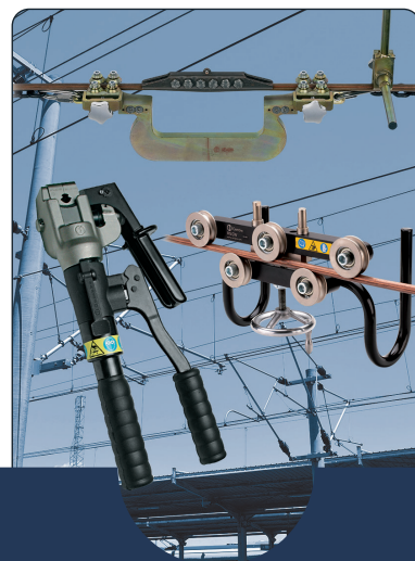
Outils pour caténaires
