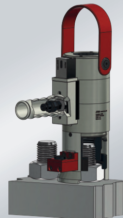
Schraubenspannzylinder
